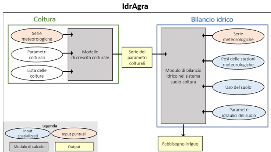
Figura 2 – Schema dei dati in ingresso e in uscita ai due moduli di calcolo di IdrAgra
